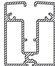
Saçak Profili Eaves Profile
