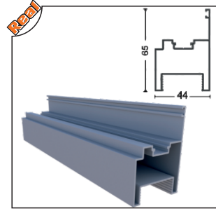
ISICM31-1016 İspanyolet Kollu Profili Espagnolette Arm Profile
