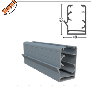
GLD-1002 Oluklu Kasa Profili Dropper Frame Profile
