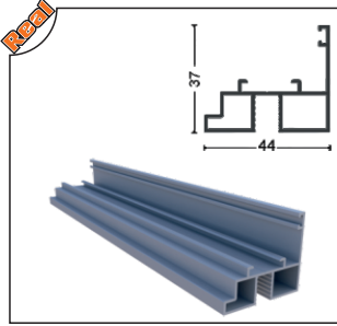
PRGLD-1009 İspanyolet Kol Profili Karşılığı 8 mm Espagnolette Arm Profile Of Opposite
