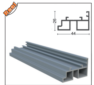
PRGLD-1006 Tıjlı Kollu Fitil Karşılığı Espagnolette Arm Opposite Seal
