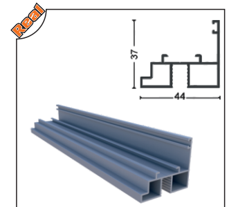
PRGLD-1009 İspanyollet Kol Profil Karşılığı 8 mm Espagnolette Arm Profile Of Opposite
