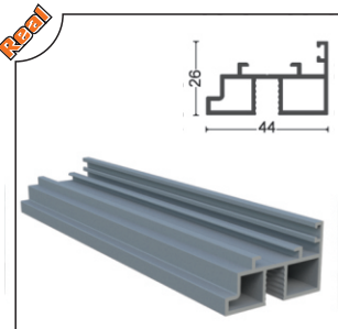
PRGLD-1006 Tıjlı Kollu Fitiil Karşılığı Espagnolette Arm Opposite Seal
