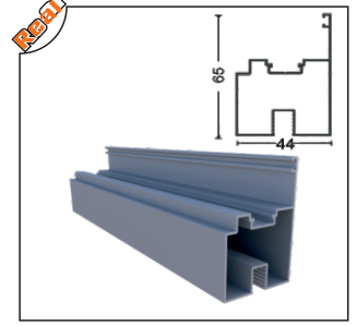
PRGLD-1008 8 mm İspanyolet Kol Profili 8 mm Espagnolette Arm Profile
