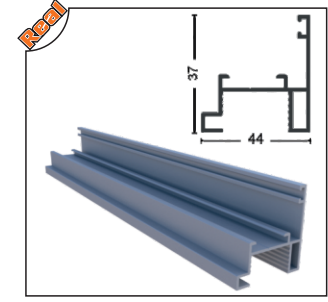
ISICM21-1010 İspanyolet Kol Profil Karşılığı Espagnolette Arm Profile Of Opposite
