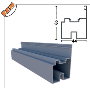
PRGLD-1008 8 mm İspanyollet Kol Profili 8 mm Espagnolette Arm Profile
