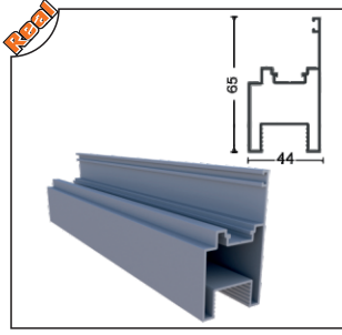
ISICM21-1009 İspanyolet Kollu Profil Espagnolette Arm Profile
