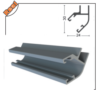
ALMFTL-1003 135 Fitol Aluminum 135 Seal
