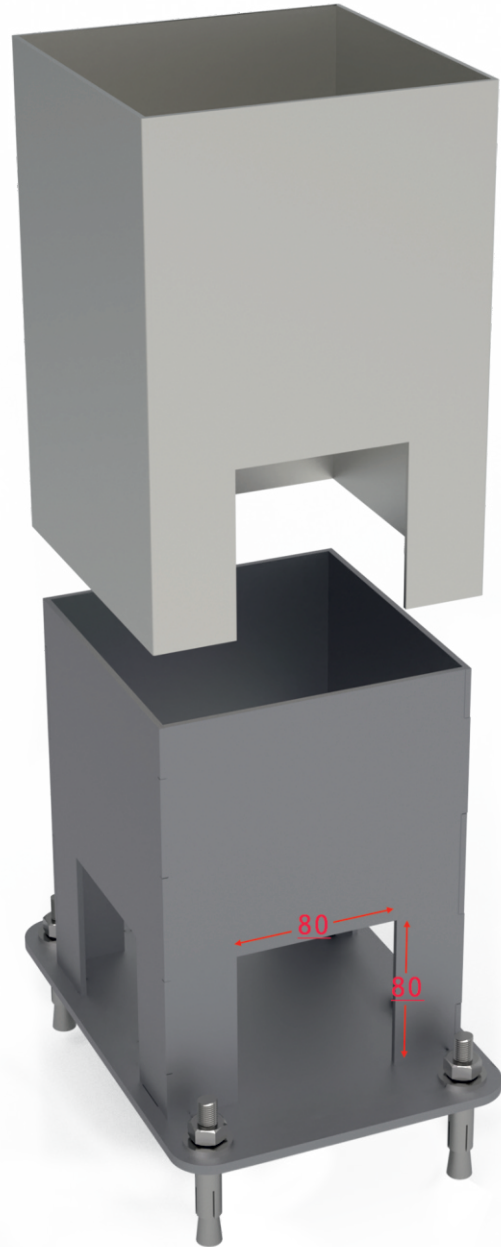
Ayak Alt Köşe Bağlantı Foot Bottom Corner Connection BIO-2519
